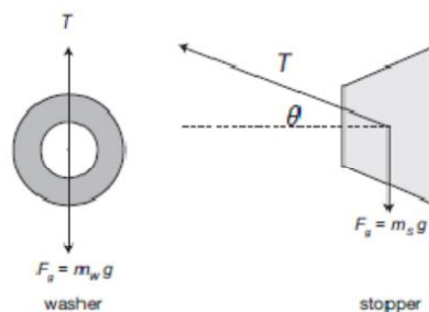
Σχήμα 2: Διανυσματικό διάγραμμα δυνάμεων
